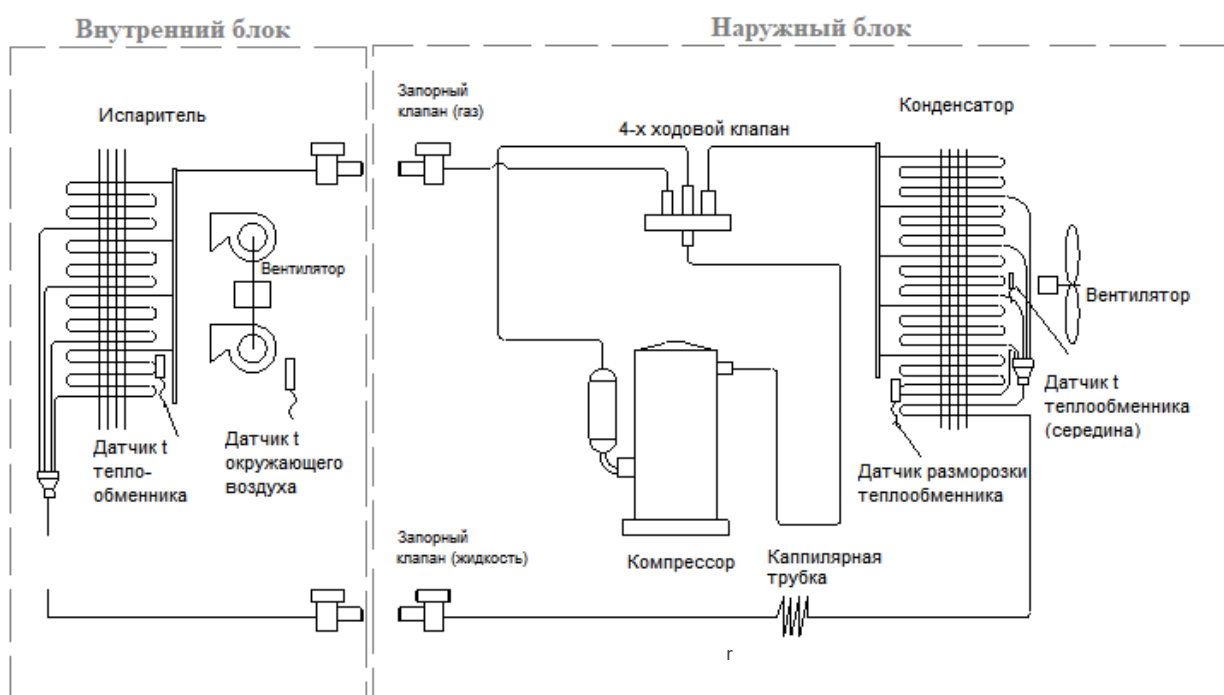
Рис.2.1-Фреоновый контур кондиционера
