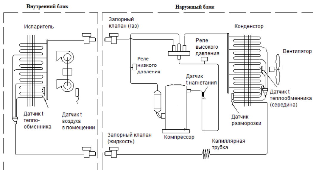
Рис.2.2 -Фреоновый контур кондиционера
